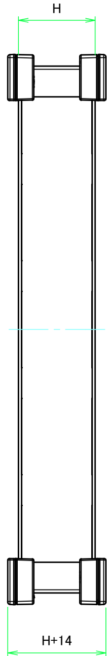
Dパネル2 / D Panel 2
