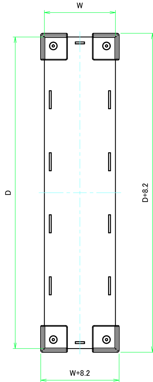
Wパネル1 / W Panel 1
