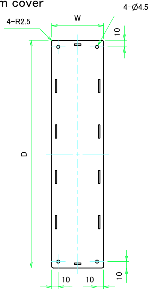
上カバー表面 / Top cover Frontside
